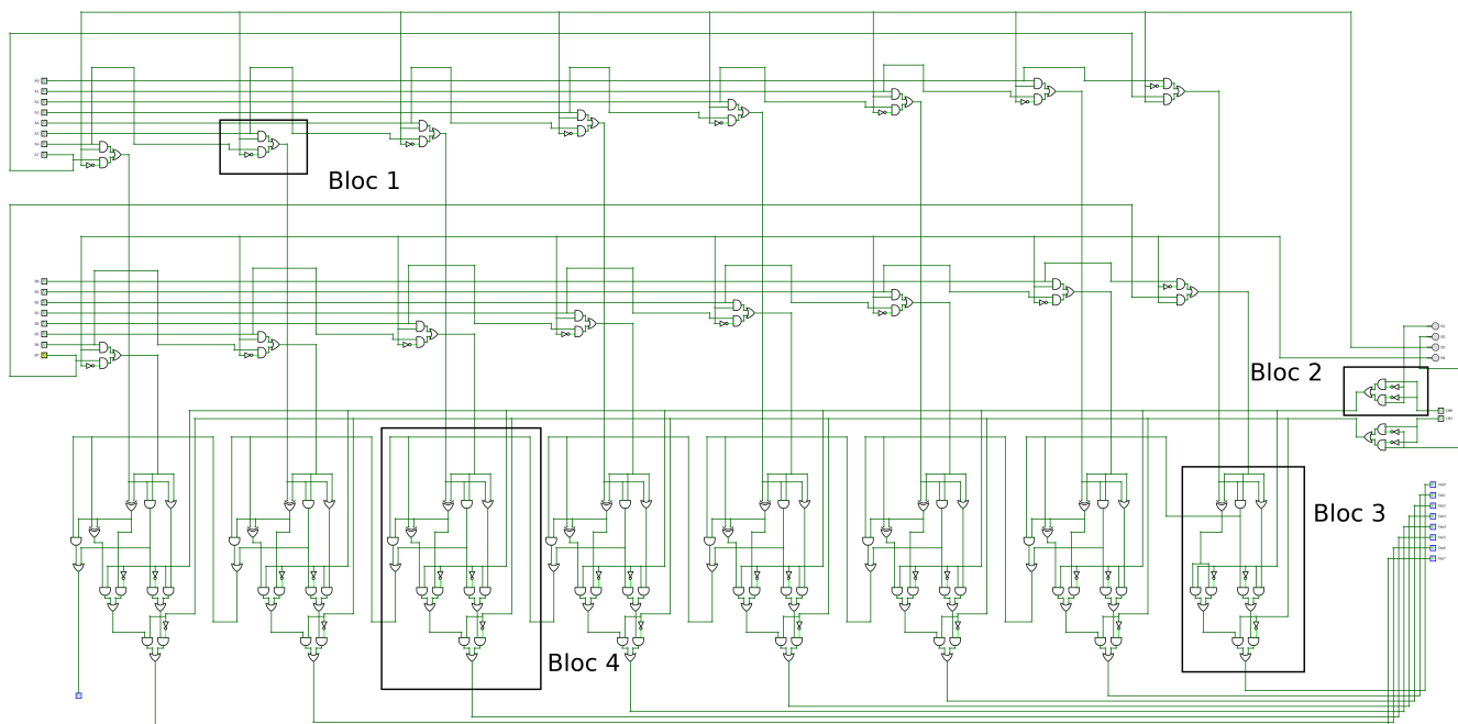
Figure 4: Les 4 blocs de portes logiques
